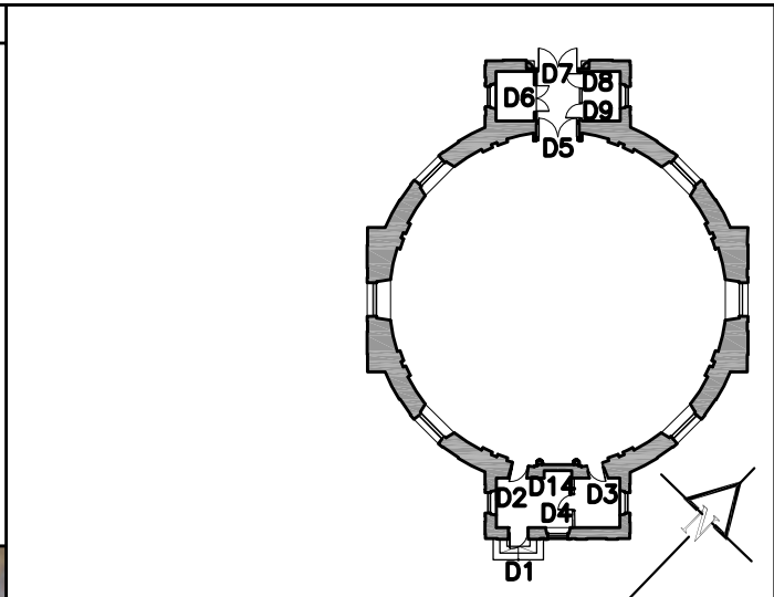
1. STĀVA PLĀNS
